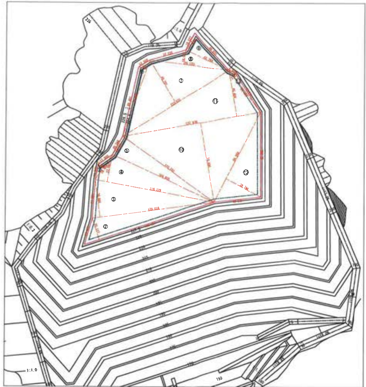
EL226.5
