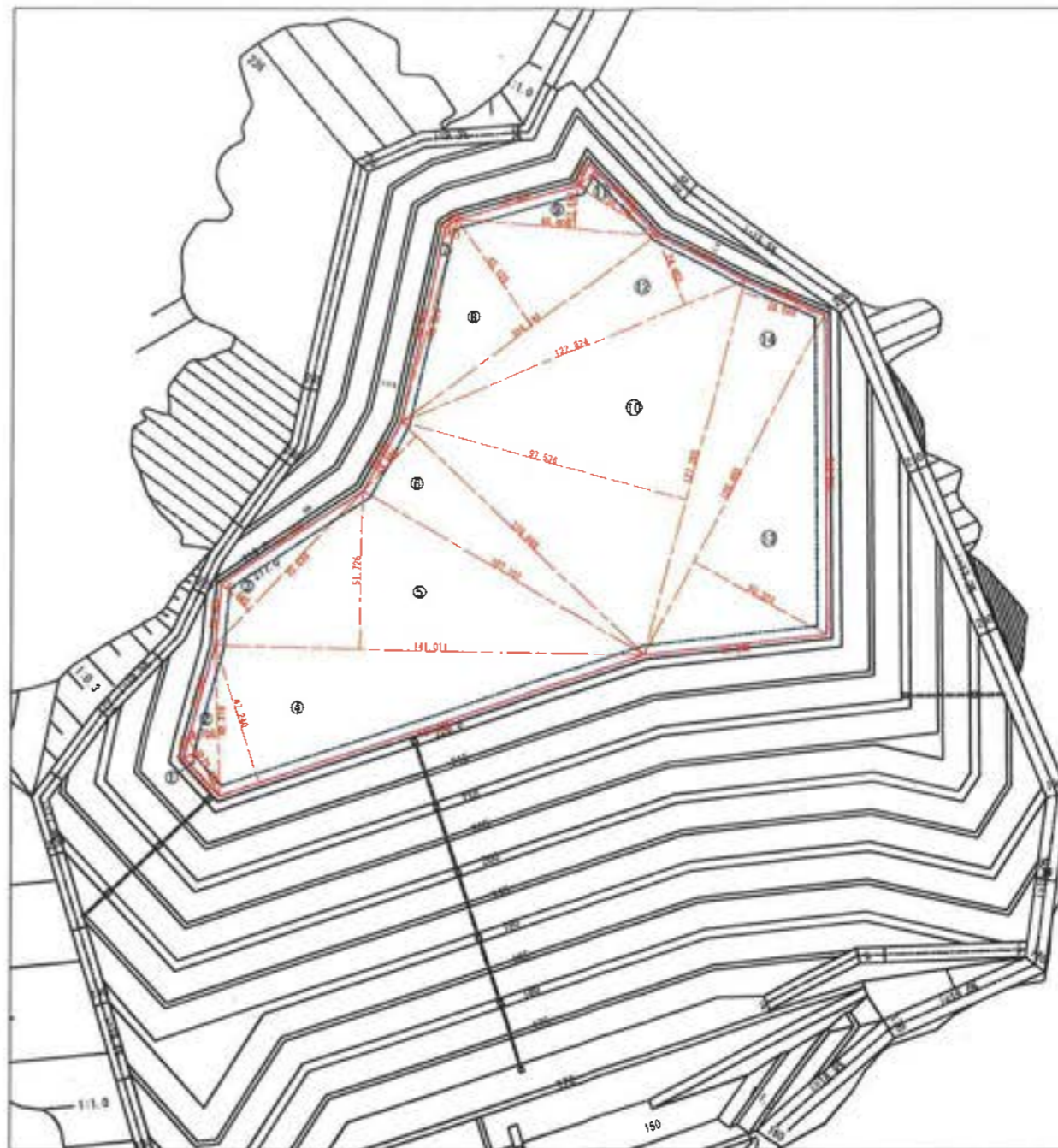
EL219.0
