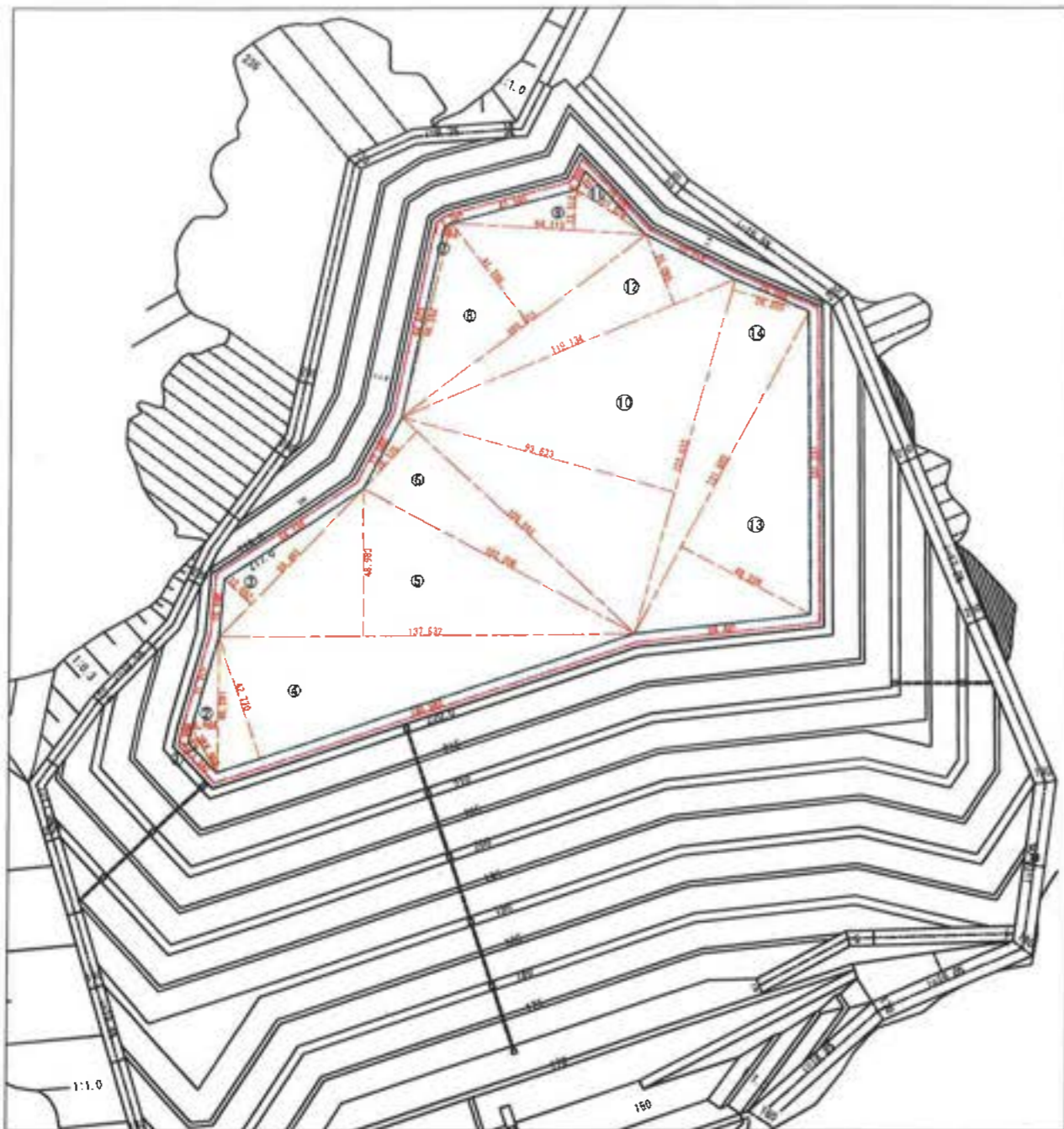
EL217.0
