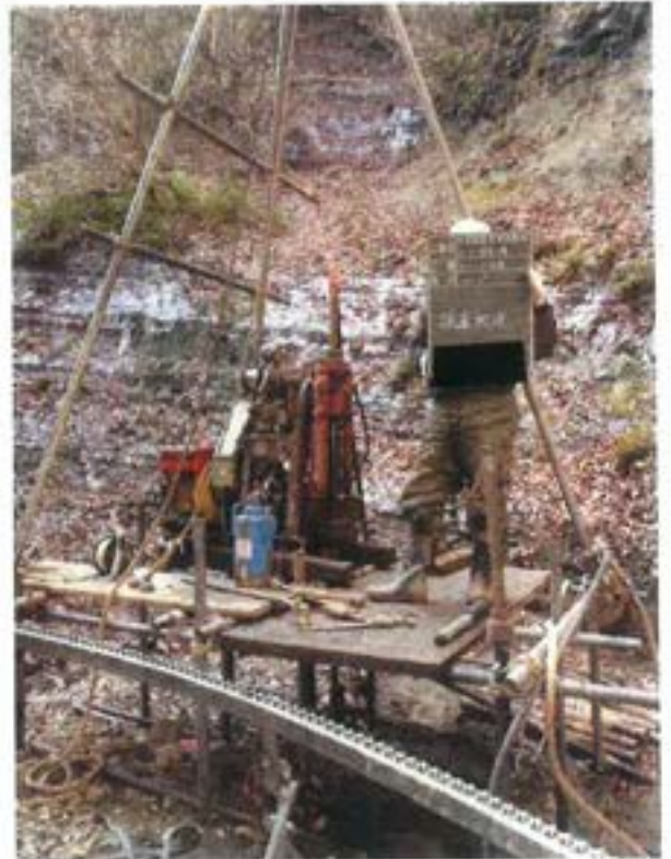
掘進状況
