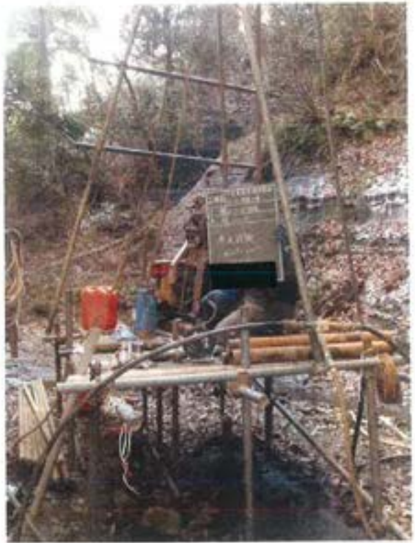
現場透水試験 4.00~6.00m
